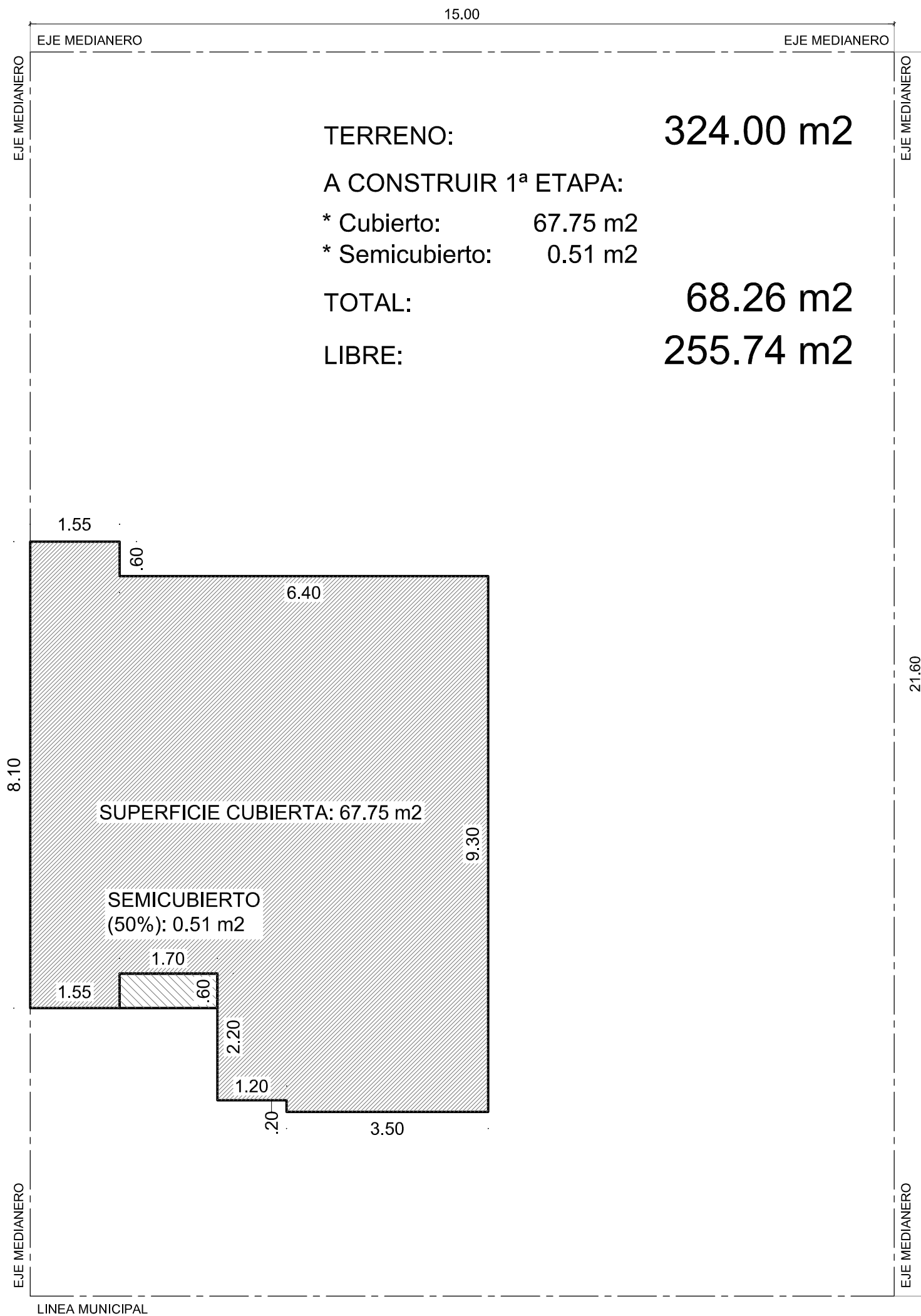
SILUETA DE SUPERFICIES / Esc. 1:100
