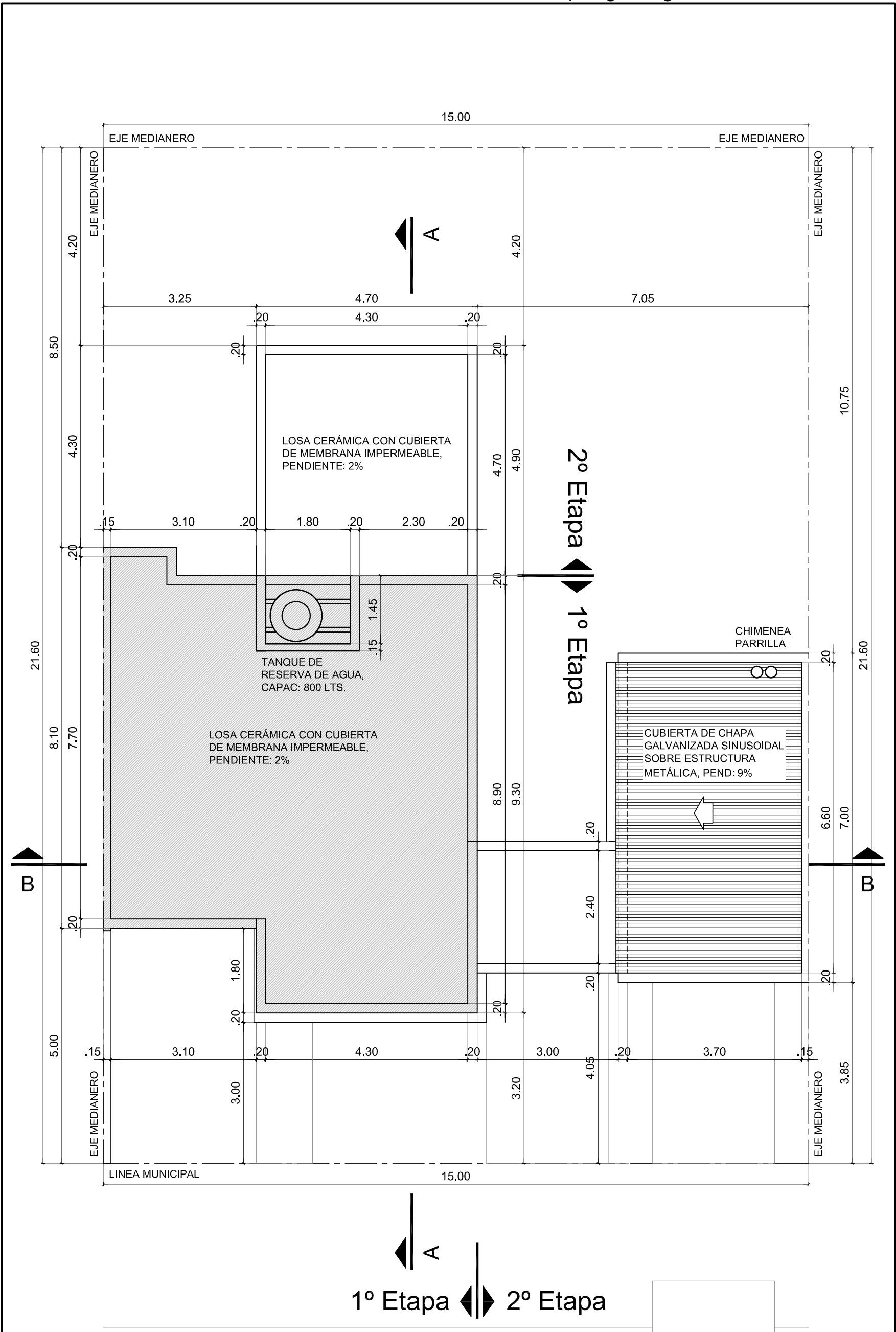
LINEA CORDÓN VEREDA PLANTA DE TECHOS / Esc. 1:100
