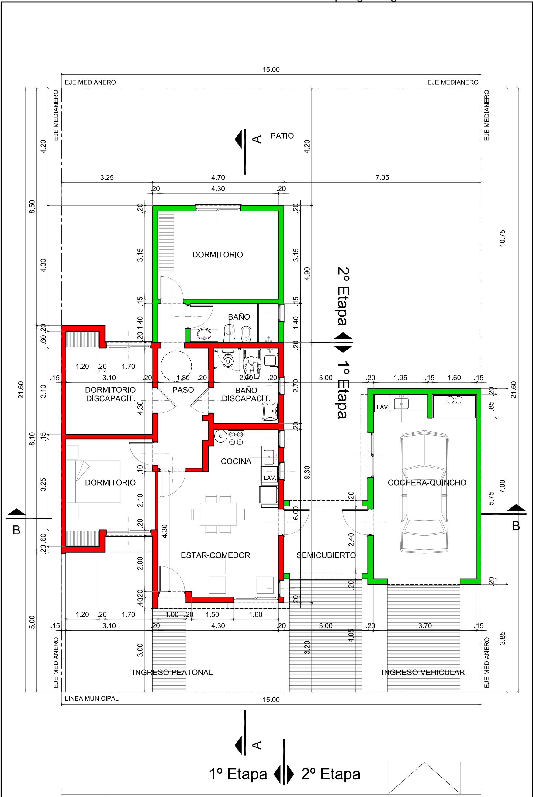
PLANTA CON FUT.AMPLIACIÓN / Esc. 1:100
