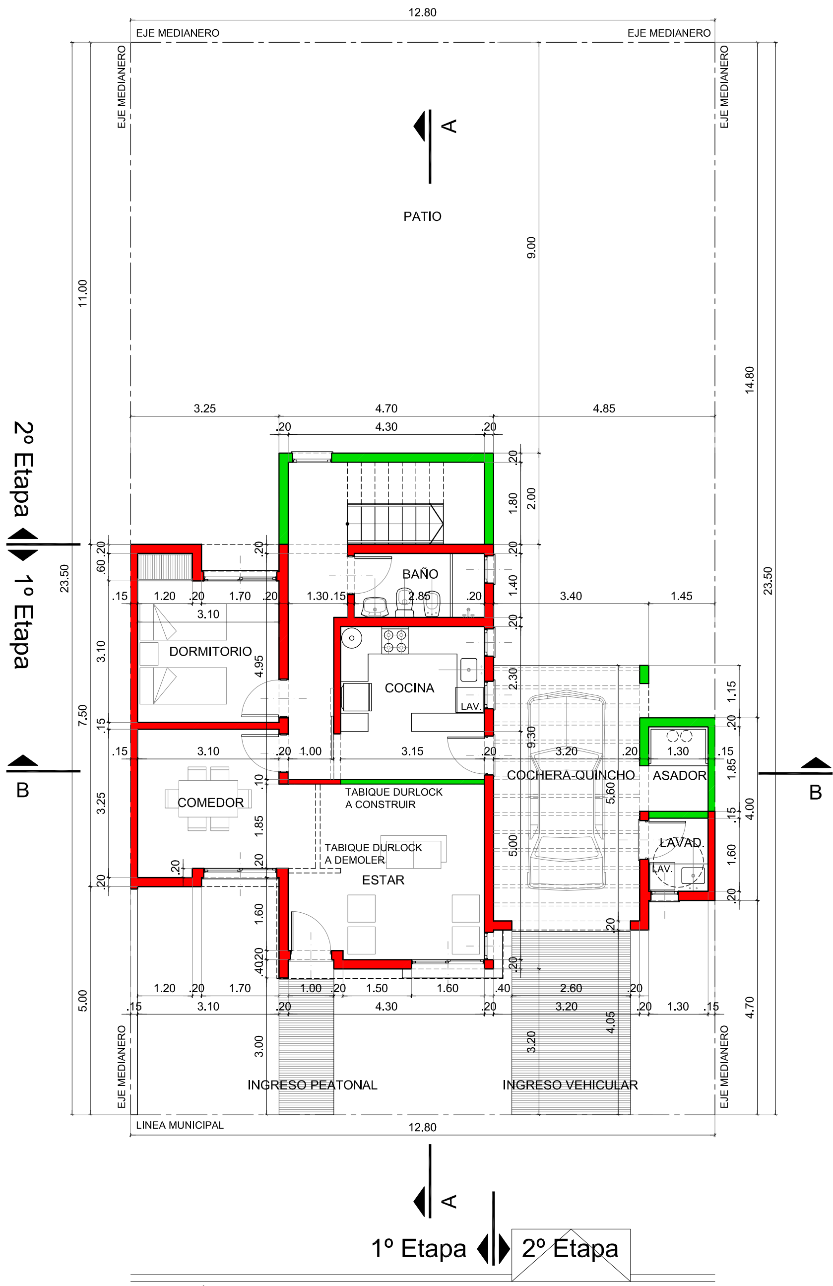
PLANTA / Esc. 1:100 CON FUT. AMPLIACIÓN EN P.ALTA
