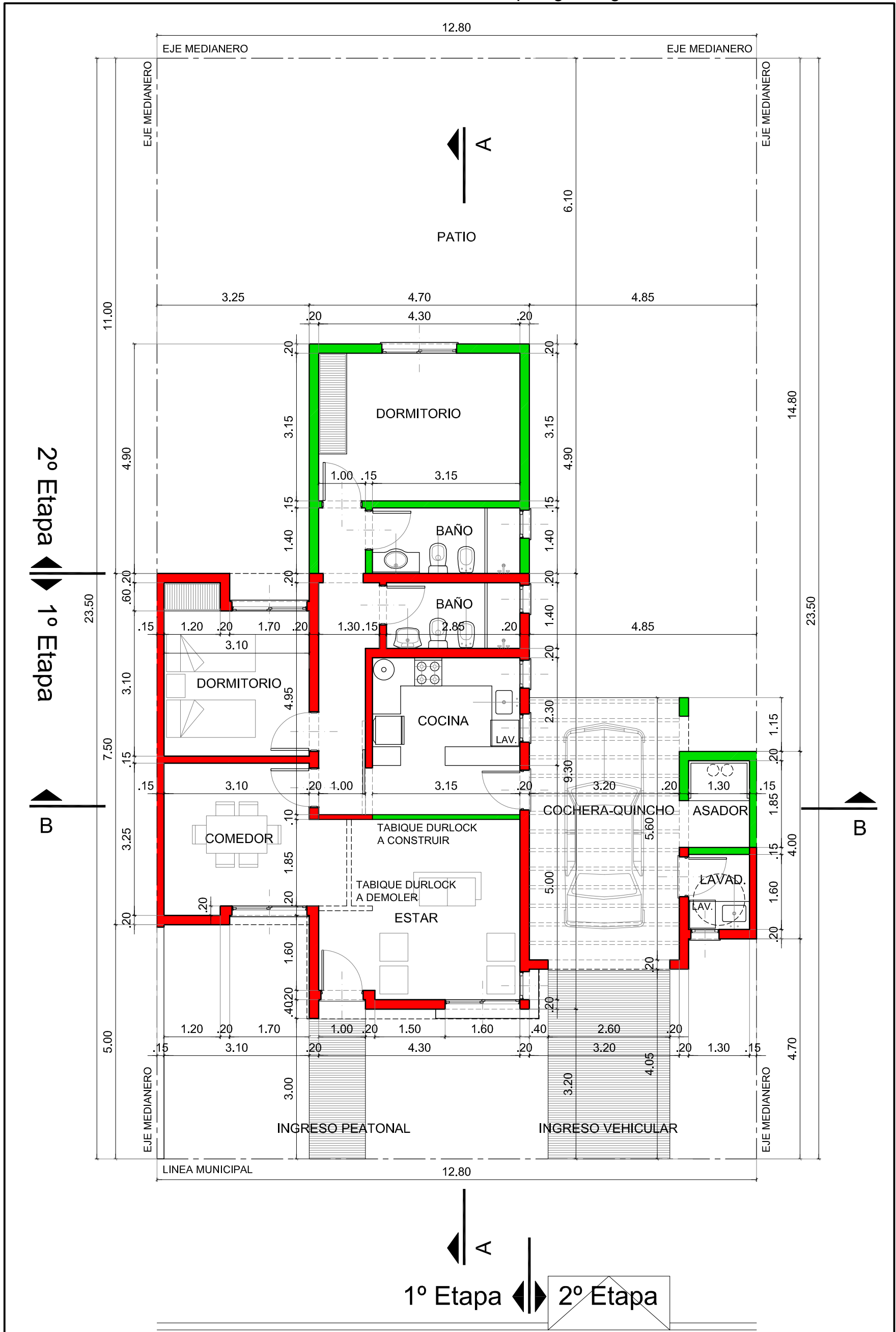
PLANTA / Esc. 1:100 CON FUT. AMPLIACIÓN EN P.BAJA
