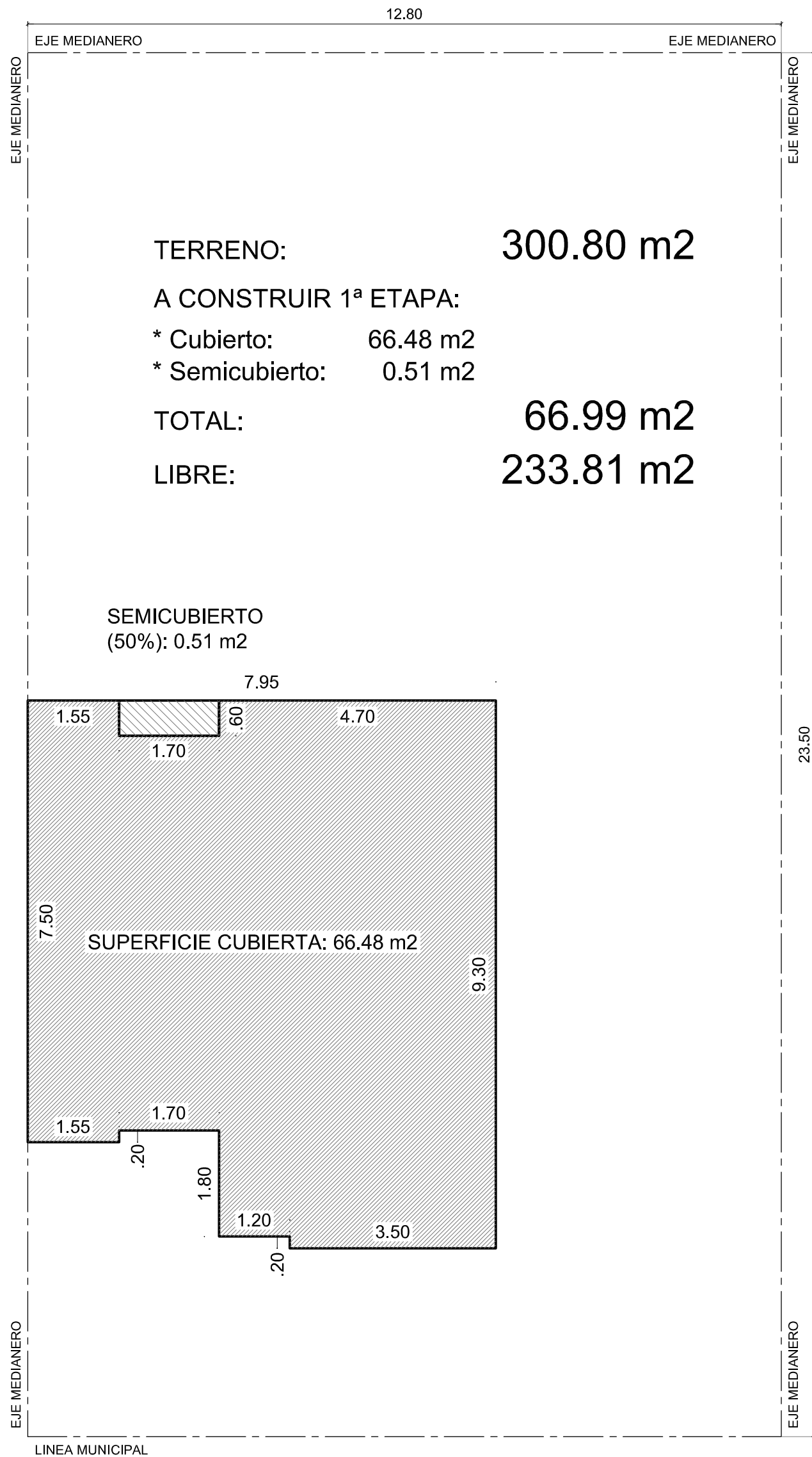
SILUETA DE SUPERFICIES / Esc. 1:100
