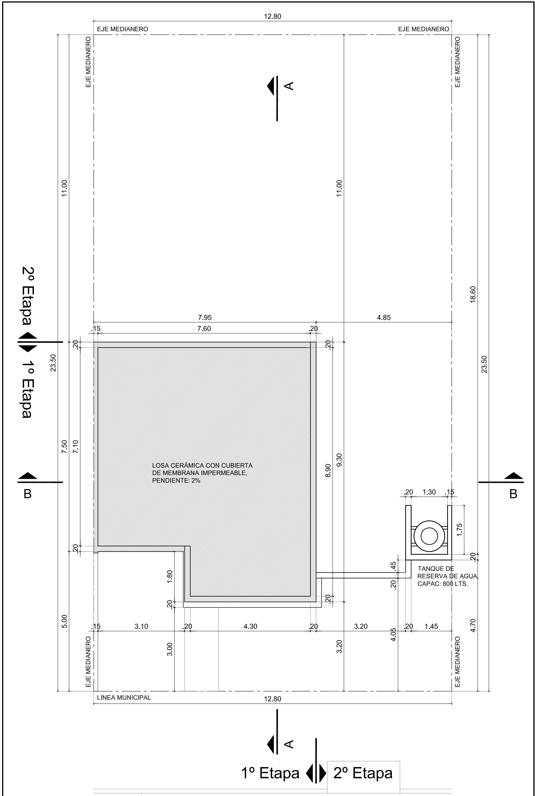
PLANTA DE TECHOS 1º ETAPA / Esc. 1:100
