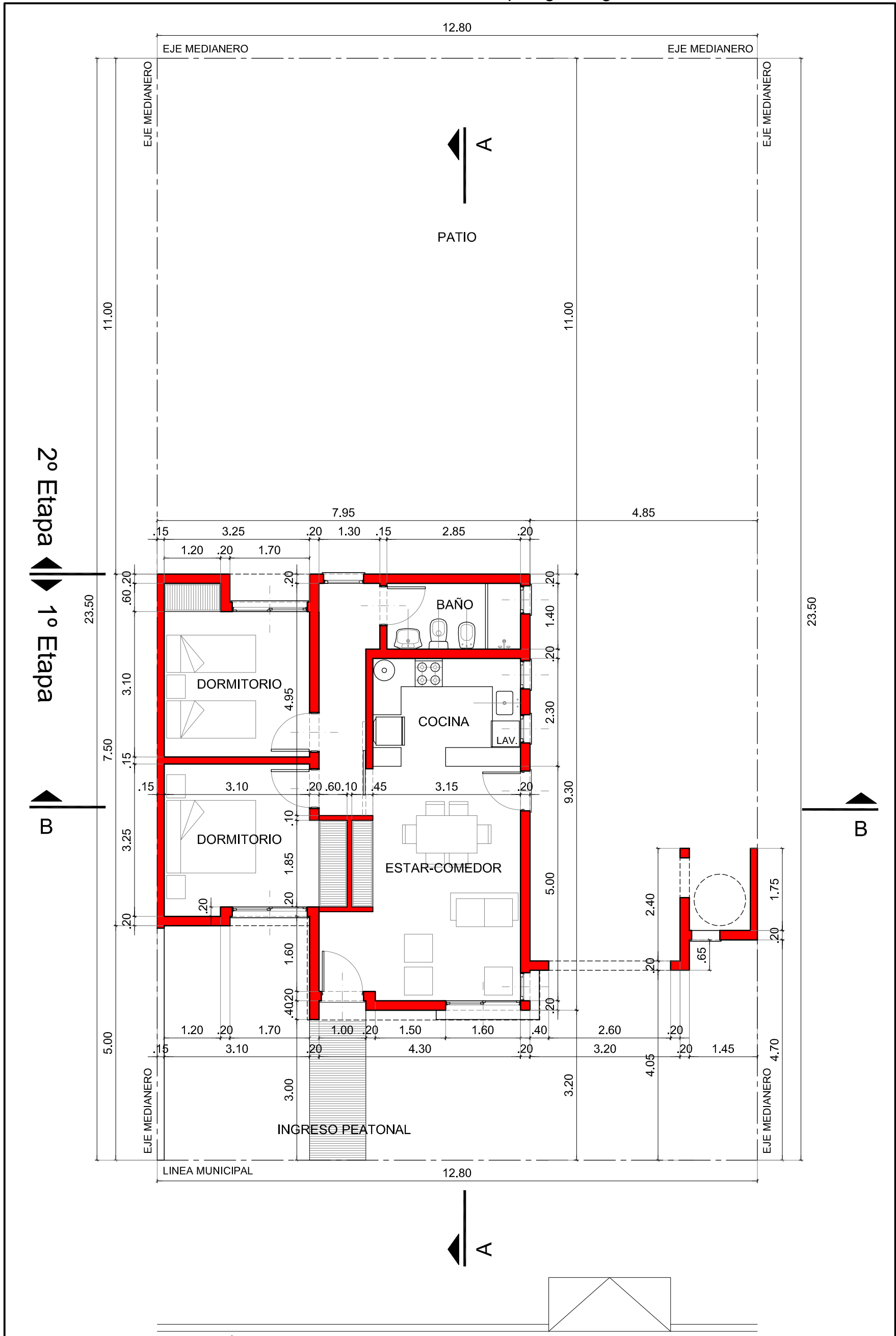
PLANTA 1º ETAPA / Esc. 1:100
