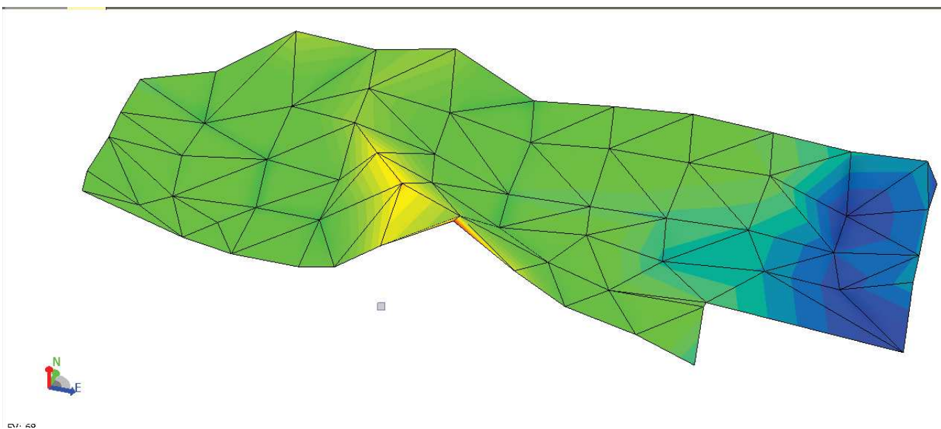
PLANO 3: MODELO DIGITAL DEL TERRENO. Se representa una figura en 3D a escala, de la superficie del terreno natural, que indica las diferentes alturas y la morfología del mismo.
